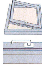
Kippstellung des Flügels
